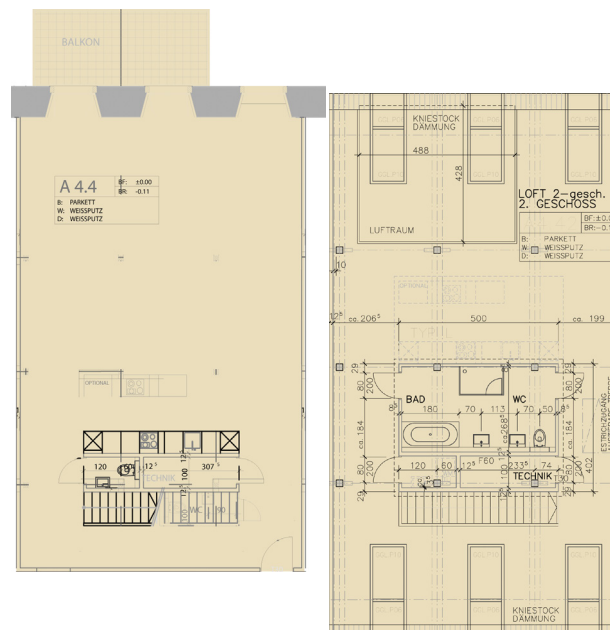
Grundriss
