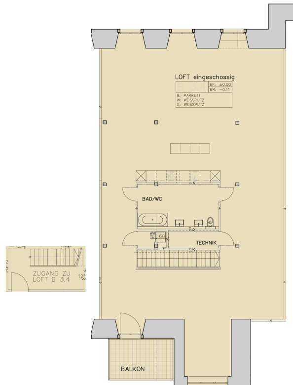
Grundriss
